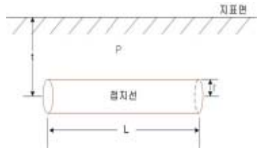
(그림2-10) 매설지선 전극의 구조 Figure 2.10 Structure of Grounding Line Electrode
