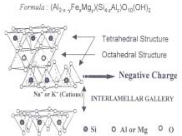
그림2-2. MMT의 구조
